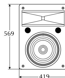
UM-100P (вид спереди)
