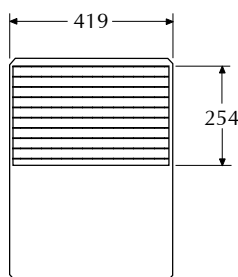
UM-P (вид сзади)
