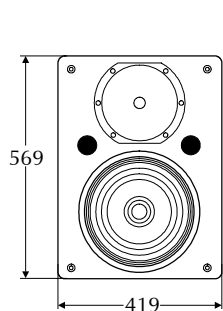
UM-1P (вид спереди)
